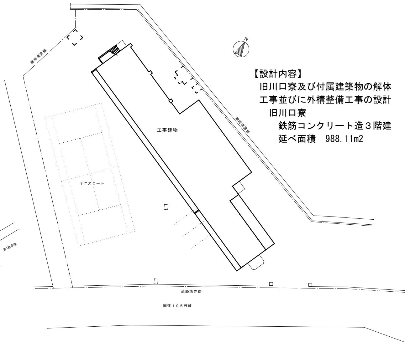
配置図 1/200
